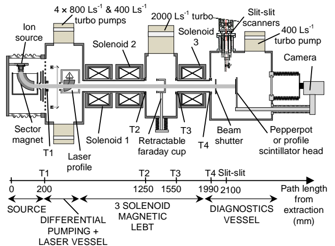
FIG 2: A schematic of the FETS LEBT beam line.
