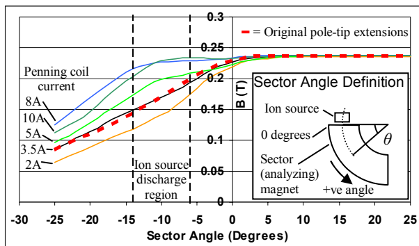
Figure 4: Magnetic survey data.
